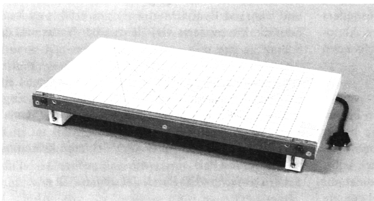
Kunststoff-Biegeapparat PA 3750 mit integriertem Netzgerät, Biegelänge 400 mm
