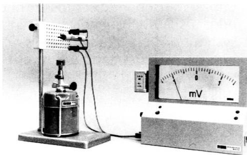
Temperatur messen mit Thermoelement PA 7295
