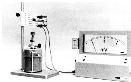
Temperatur messen mit Thermoelement PA 7295 siehe «Physik für Sek I» Seite 144 (PA 150)
