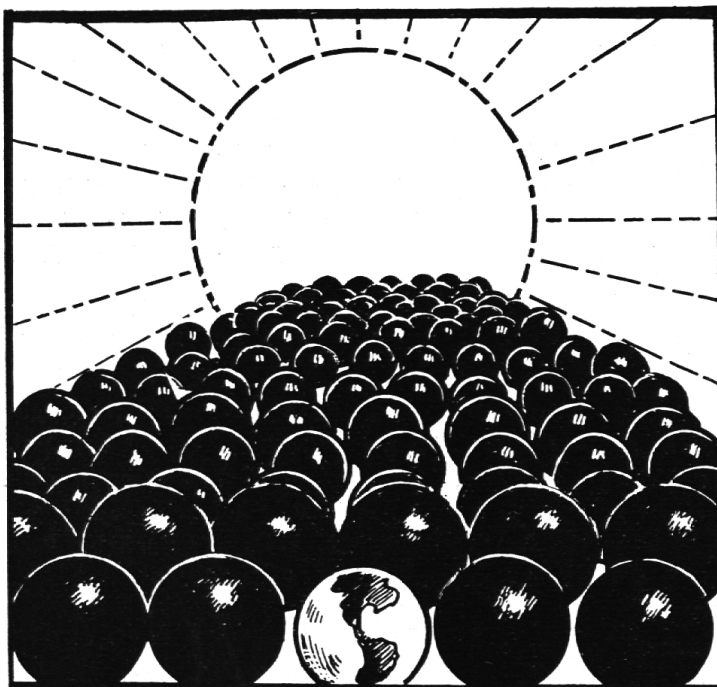
Um die von der Sonne ausgestrahlte Wärme zu erzeugen, müßte man jährlich 90 Erdkugeln aus bestem Anthrazit im »Sonnen-Ofen« verbrennen – Zwei Darstellungen zum Artikel »Von Sonne, Mond und Sternen« (mit 24 Bildern)
