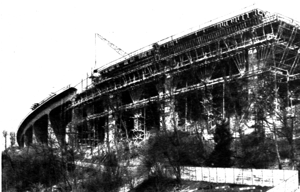
Los 2: Bau des Viaduktes über die Talwegmulde, links fertiger Teil, rechts Gerüste mit Turmdrehkran.
