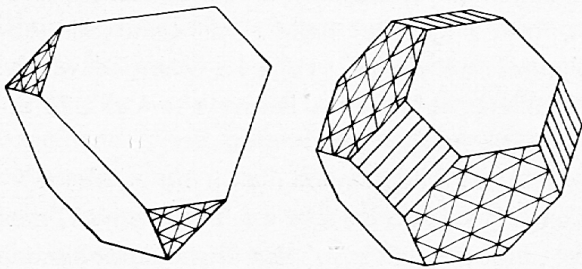
Fig. 11. Fahlerz und Zinkblende.
