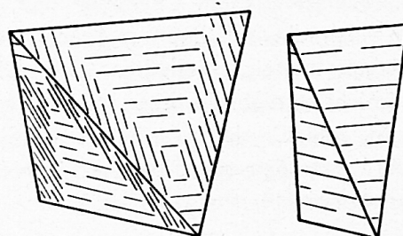
Fig. 14. Kupferkies (bisphenoidisch).
