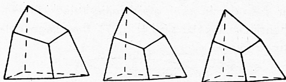
Fig. 8. Verschiedene Deltoidikositetraeder (Granat vom Lolenpass, Mittaghorn-Saastal, Gotthard).
