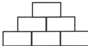
Abb. 3: Zahlenmauern: «Auf je zwei benachbarte Steine einer Schicht wird ein dritter Stein gesetzt, in den die Summe der beiden unteren Steine einzutragen ist»
