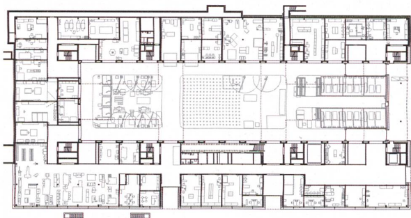
Grundriss Hallengeschoss (Ebene E).
