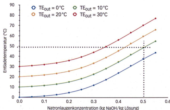
Die Entladetemperatur hängt von der Verdampfungstemperatur (Temperature Evaporator = TE_{out} ) und der Natronlaugenkonzentration ab. Bei einer 50-%-igen Lösung und TE_{out} = 10^\circ\text{C} beträgt die Entladetemperatur 48°C.
