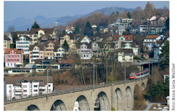
Titelbild Die Instandsetzung des 296 m langen Glattalviadukt in Herisau gehört zu den grösseren und augenfälligsten Teilprojekten des «Cluster 2012»
