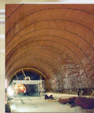
DELTA-MS 20 Zuverlässige Drainageeigenschaften im Tunnelbau
