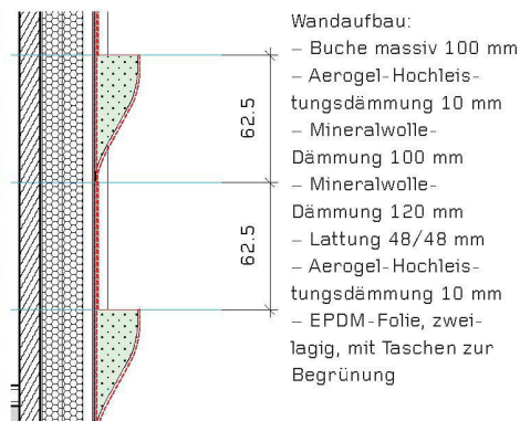
01–02 Prototyp der mit Winterjasmin bepflanzten Folienfassade am «Woodstock» auf der Swissbau 2010 (Foto: Contec; Plan: Artevetro Architekten)
