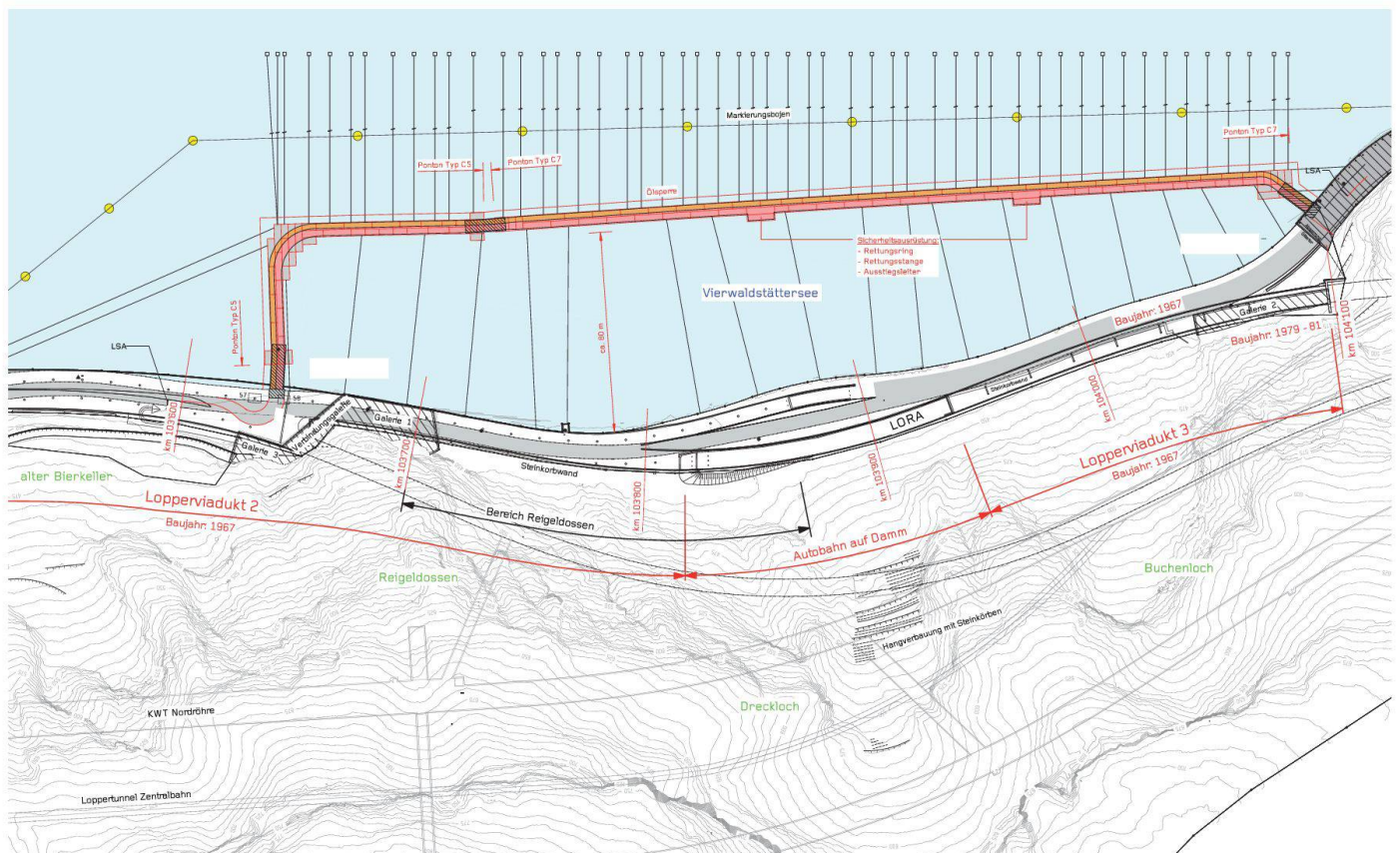
03 Situation im Gebiet Lopperviadukt 2 mit Reigeldossen und der Ponton-Notbrücke (Plan: Slongo Röthlin Partner AG, Stans)
