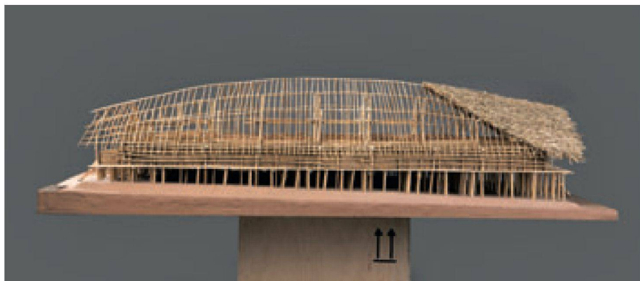
01+02 Modell und Konstruktionsdetail: Langhaus der Kaluli aus Papua-Neuguinea. Die Häuser sind durch die Sippe gemeinschaftlich aus roh belassenen Stämmen erstellt, mit Lianen verkleidet und von bis zu 60 Personen bewohnt. Es handelt sich um grosse Einraumhäuser auf Stelzen. So werden Schäden aus Überschwemmungen vermieden, und die Konstruktion ist ringsum effizient belüftet (Fotos: vinipphoto, Virginie Otth und Nicolas Lieber)
