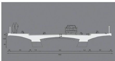
07 «Houdini»: Die Brücke besteht aus einem zweistegigen vorgespannten Plattenbalken mit schlanken, nach innen geneigten Stegen. Die Trägerhöhe nimmt in den Seitenfeldern linear gegen die Pfeiler hin zu, im Mittelfeld ist sie parabolisch überhöht. Die Pfeiler sind im oberen Teil Y-förmig aufgelöst
