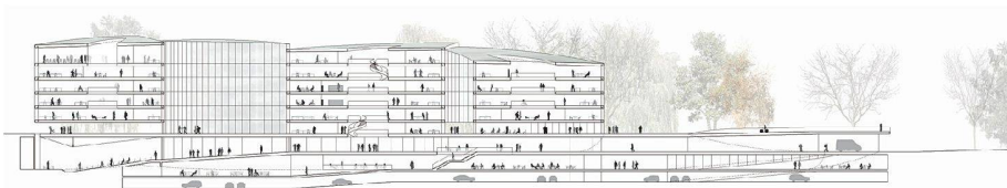
04 Längsschnitt
