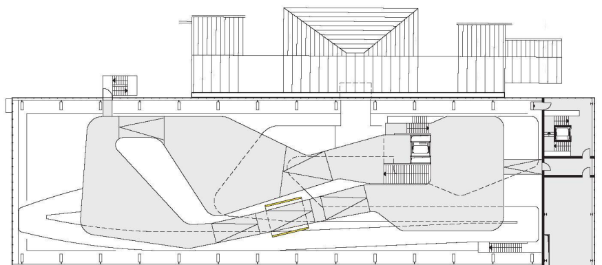
04 Quer-, Längsschnitt und Grundrisse Niveau 1 und 3, Mst. 1:700 (Pläne: Gatermann + Schossig)
