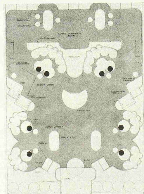
Entwurf von Hans Brüttsch, Zürich, Grundriss
