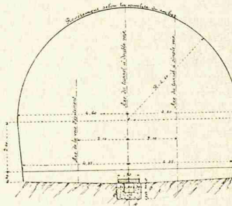
Nr. 6. An der Ausweichstelle (Tunnelmitte).
