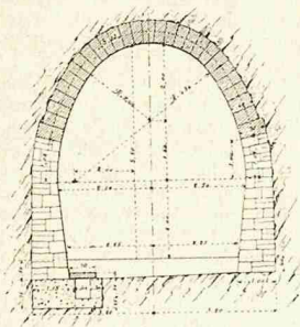
Nr. 4. Im Gebirge mit grossem Vertikaldruck.
