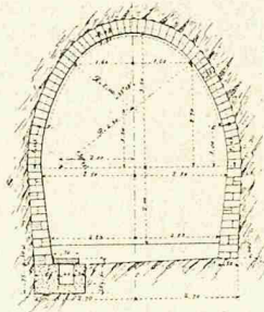
Nr. 5. Im Gebirge mit grossem Seitendruck.
