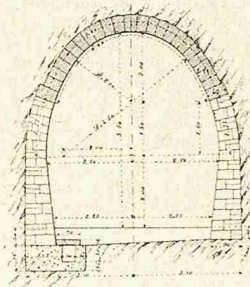
Nr. 6. An der Ausweichstelle (Tunnelmitte).
