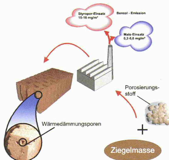
Die Backsteinherstellung: Porosierungsmittel verbessern die Dämmwirkung des Produkts, entwickeln beim Brennvorgang aber meist toxische Abgase. Maisstärkehaltige Porosierungsmittel sind dagegen emissionsarm (Bild: Frank Reckert, Institut für Kunststofftechnik)
