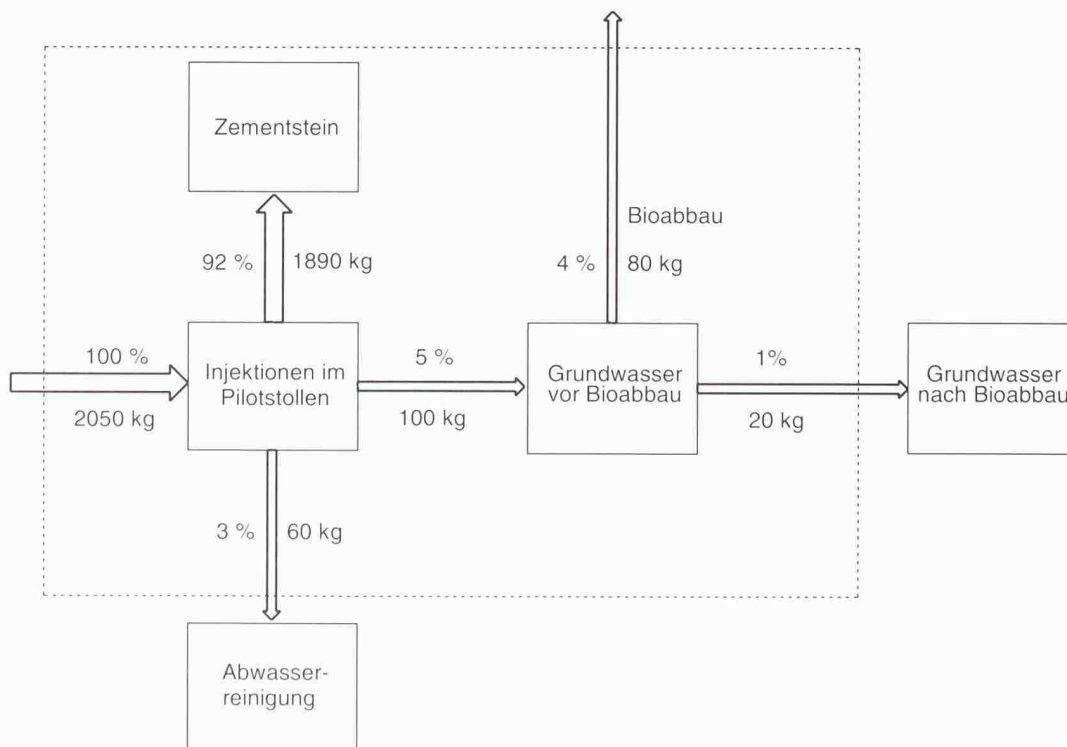
4 NSFK-Massenflüsse der SBB-Tunnelbaustelle 2. Doppelspur Zürich–Thalwil in absoluten Mengen und in Prozent der total eingesetzten Menge an NSFK (Bild Sabine Ruckstuhl)
