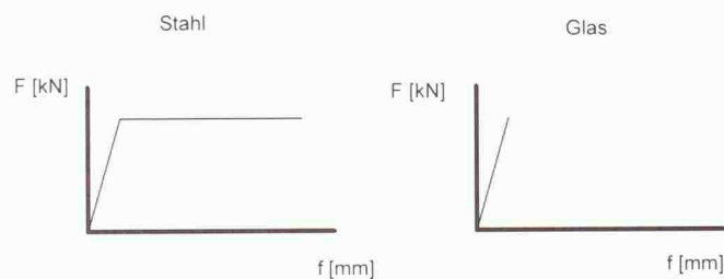
4 Spannungs-Dehnungs-Diagramme
