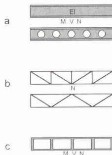
Biegesteife Systeme: (a) Biegeträger, (b) Fachwerkträger, (c) Vierendeelträger
