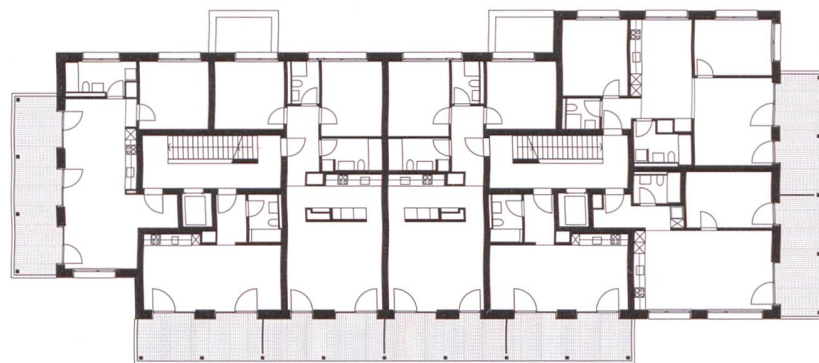
3 Erstes Obergeschoss im westlichen Längsbau | Etage supérieure de la barre ouest. | Pianta del primo piano dell'edificio a ovest, 1:400
