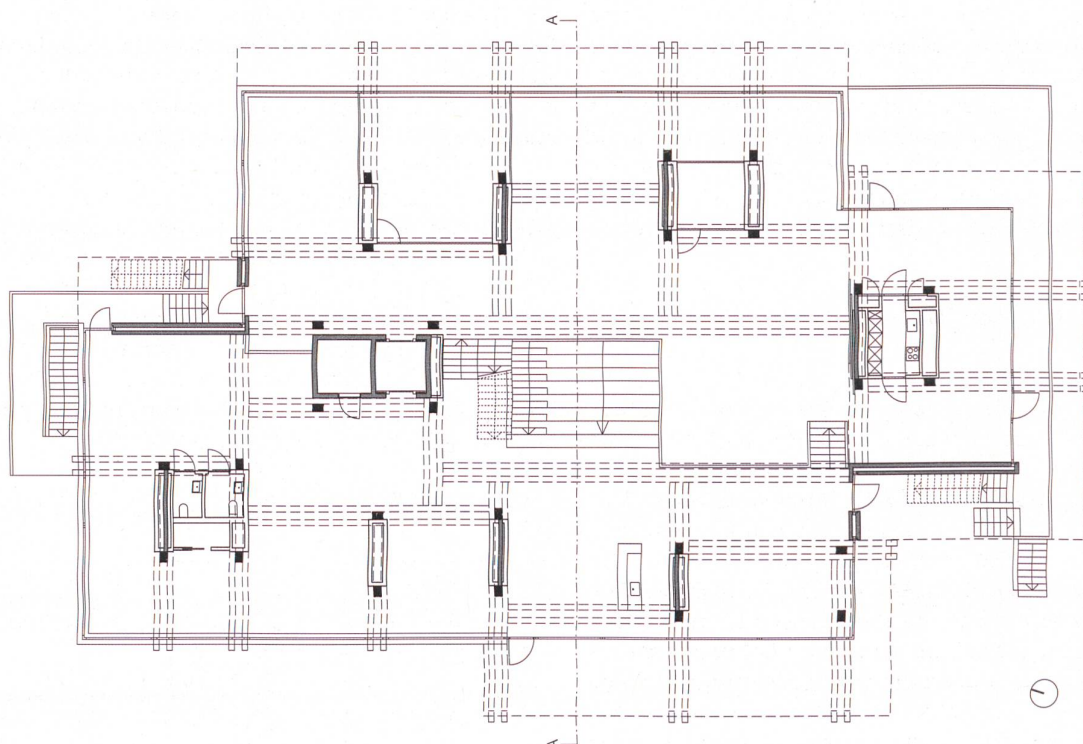
Der Grundriss des Gartengeschosses zeigt die Raum-, Trag- und Technikstruktur in der offenen Bürolandschaft.
