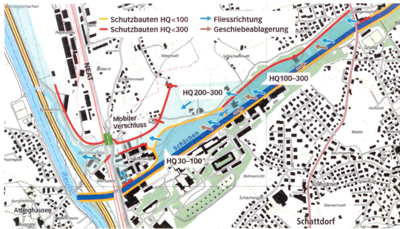
Die Ausbreitungswege bei Hochwasser «Schutzziel HQ<100» und «Überlastfall HQ<300».
