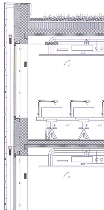
Die innere Schicht der Fassade ist effizient und unaufgeregt. Die aussen liegende Schicht aus Klarglas verschleiert die Geschosse und hebt den Grad der Abstraktion. Fassadenschnitt im Mst. 1:80.
