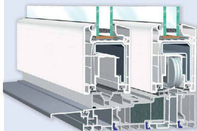
VEKASLIDE Hebe-Schiebetür
