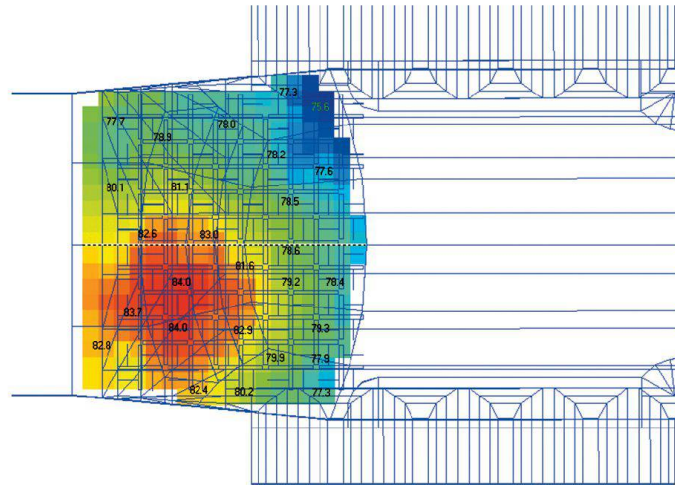
Schallintensitäten über der Bühne bei einem Konzert in der Tonhalle St. Gallen.
