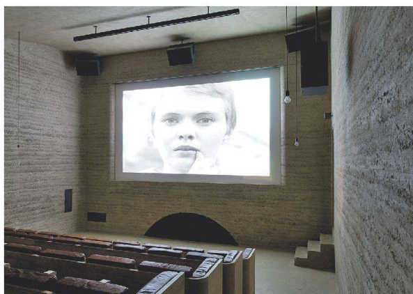
Im Kino von Ilanz (Capaul & Blumenthal Architects) treffen sich Graubünden und Vorarlberg: Stampflehm von Martin Rauch.
