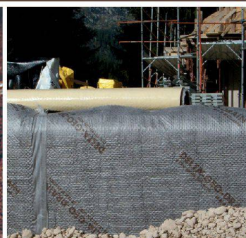
DELTA®-GEO-DRAIN Quattro Verlagiges Schutz- und Drainage- system für Dickbeschichtungen
