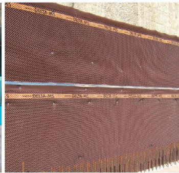
DELTA®-MS Sauberkeitsschicht, Grundmauer- schutz, Sickerschicht
