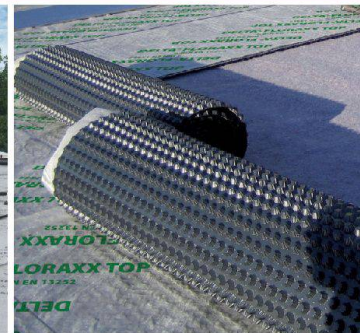
DELTA®-FLORAXX TOP Schutz-, Filter- und Sickerschicht zur Extensiv- und Intensivbegrünung
