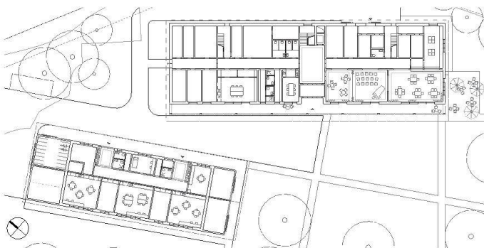
03 + 04 «Philemon & Baucis» (Bienert Kintat Architekten): Grundrisse EG und 1. OG, Mst. 1:1000. Das flache Werkhaus liegt vor dem Haupthaus in Mischbauweise mit zwei Wohntagen. Die attraktive zentrale Erschliessung bedingt zwei seitliche Fluchttreppen (Visualisierung + Pläne: Verfasser)
