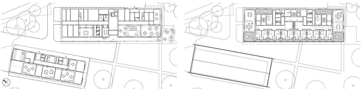
03 + 04 «Philemon & Baucis» (Bienert Kintat Architekten): Grundrisse EG und 1. OG, Mst. 1:1000. Das flache Werkhaus liegt vor dem Haupthaus in Mischbauweise mit zwei Wohnetagen. Die attraktive zentrale Erschliessung bedingt zwei seitliche Fluchttreppen (Visualisierung + Pläne: Verfasser)
