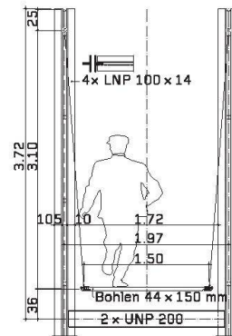
17–19 Aus in der dritten Runde: «Seilschaft» (Schnetzler Puskas Ingenieure): Der Gehweg der Hängebrücke ist mit einer Netzkonstruktion an den Hauptkabeln befestigt, an einem höher und straffer gespannten Kabel sind die systemkonformen Brüstungen befestigt. Der Bunker dient als Widerlager. Längsschnitt, Mst. 1:600; Querschnitt Stütze, Mst. 1:80
