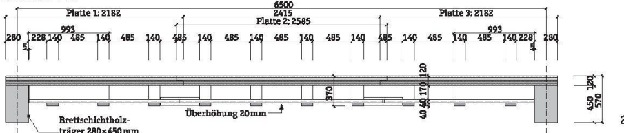
Schnitt B-B
