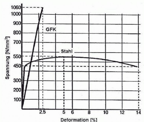
01 Typisches Spannungs-Verformungsverhalten eines GFK-Stabs und eines Stahlstabs (Bild: Rockbolt Systems AG Rapperswil)
