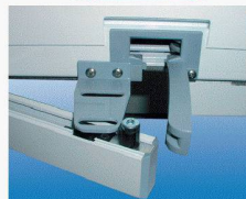
Spaltlüftung mit 2 Stufen
