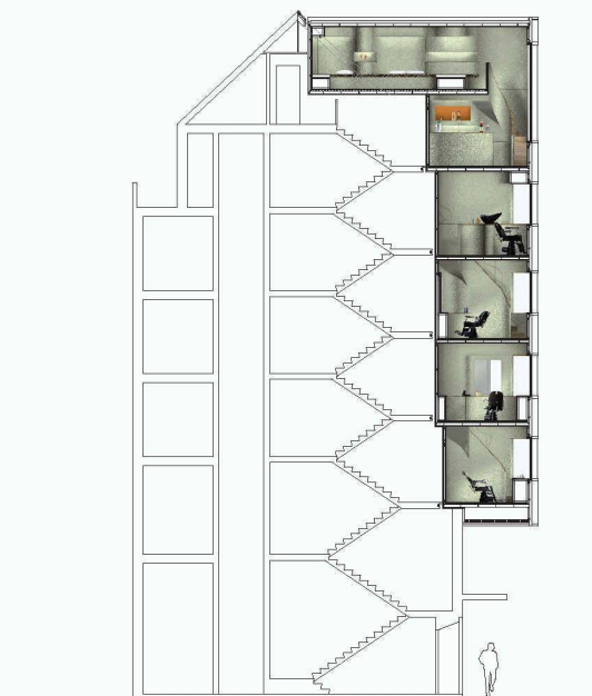
Schnitt mit dem Wand- aufbau gegen aussen
