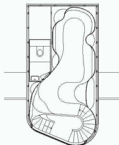
Grundriss Niveau 6: Lounge / Toilette
