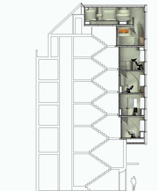
Schnitt mit dem Wand- aufbau gegen aussen
