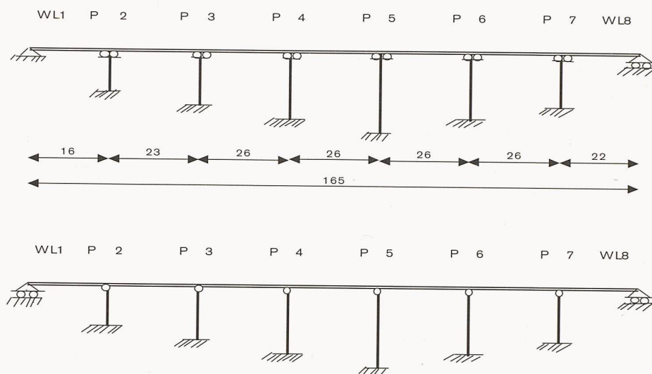
Statisches System der bestehenden (oben) und der seismisch gesicherten Chritzi-Brücke
