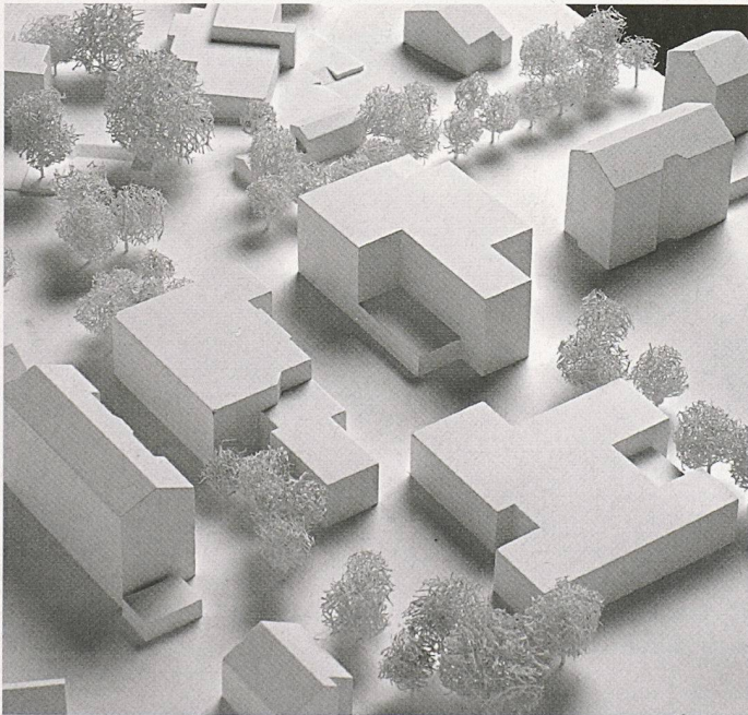
Neubau für die Fachausbildung: zu den 2 bestehenden Schulbauten einen eigenständigen dritten (oben) hinzugefügt (1. Rang, bonnard / wœffray)
