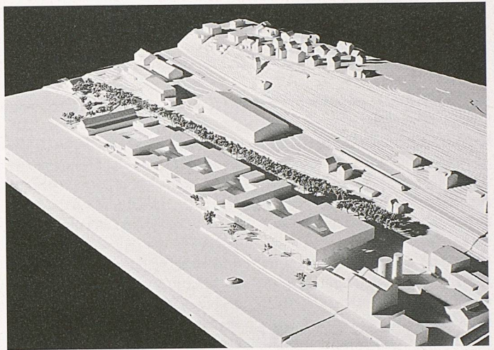
Zwischen den zwei Reihen ein langgezogener Innenhof (3. Preis, Weisser Architektur & Bau)
