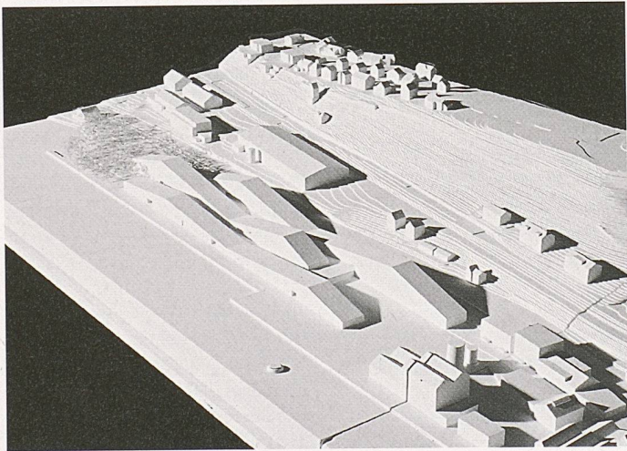
Die grossen geneigten Dächer der 3 Baukörper erlauben auch von den hinteren Bauten einen Blick auf den See (4. Preis, Schmid Kuepfer Architekten)
