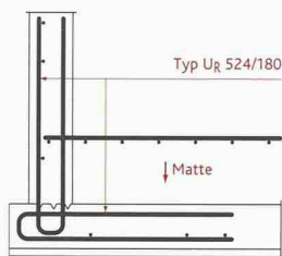
Anschlussbewehrung Bodenplatte-Wand
