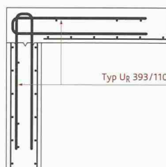
Anschlussbewehrung Wand-Decke
