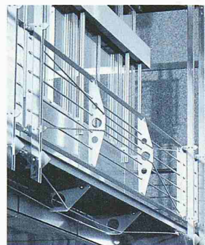
Winkel gleichschenklig
