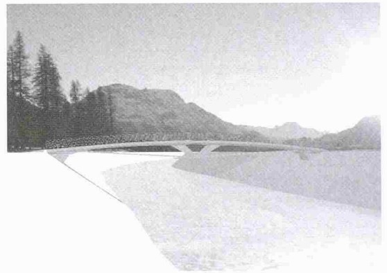
1. Rang Flazbrücken Samedan: Perspektive und Längsschnitt (Mst. 1:500) für den Standort Gravatscha von Ingegneri Pedrazzini und Baserga Mozzetti architetti. Für die ständigen Lasten funktioniert die Struktur als Bogen mit Zugbändern. Die Diagonalen verleihen der Fahrbahn die erforderliche Steifigkeit zur Aufnahme der variablen Lasten. Material: Beton, Zugbänder und Diagonalen vorgespannt (Bilder Projektverfasser)
