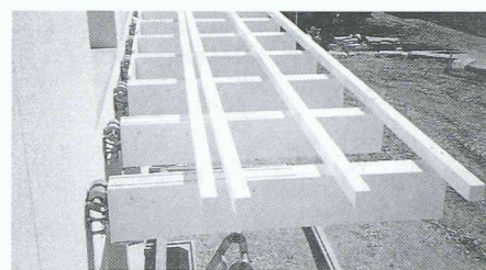
Wärmegeprägter Kragbalken aus Holz. Sichtbar sind die Einhängezughaken und die bereits vorbereitete Queraussteifung der Balkonplatte (Bild: Schöck-Bauteile AG)
