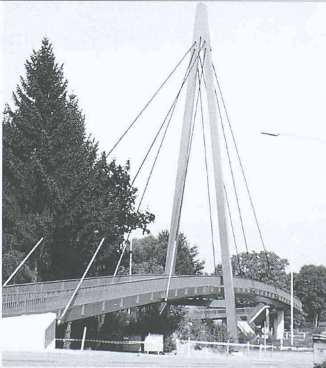
Projekt: Schrägseilbrücke Rümliang Ingenieure: Emeh & Berger AG, Zürich
