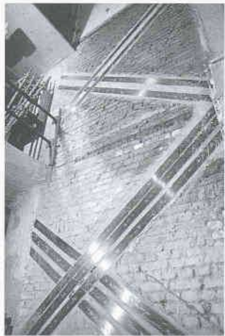
5 Anordnung der CFK-Lamellen auf der Mauerwerktragwand
