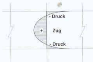
Spannungsverteilung im Querschnitt durch eine thermisch vorgespannte Glasscheibe
