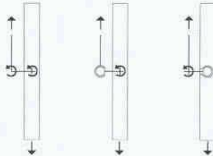
Arten der Glasbefestigung: Starre Auflagerung, Gelenk ausserhalb der Glasscheibe, Gelenk innerhalb der Glasscheibe
