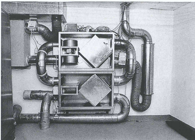
Das Lüftungsgerät ohne Abdeckungen. Die beiden hintereinandergeschalteten Wärmetauscher sind deutlich zu erkennen
