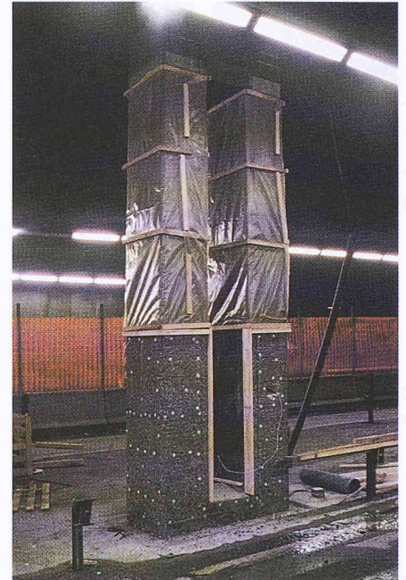
Bild 5. Doppelstütze mit KKS
