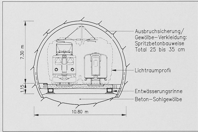
Bild 4. Normalprofil Zweispurttunnel im Flysch
