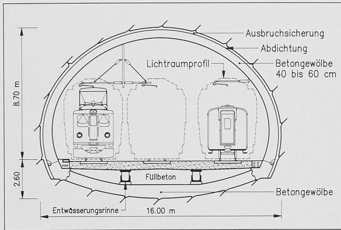
Bild 3. Normalprofil Dreispurttunnel
