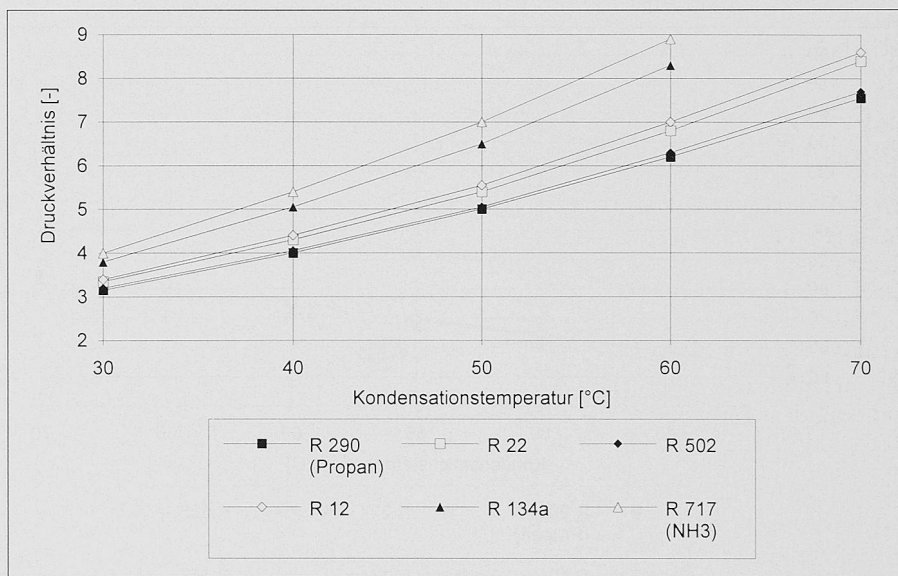
Bild 2. Druckverhältnisse, Verdampfungstemperatur, t_0 = -10^\circ\text{C}
