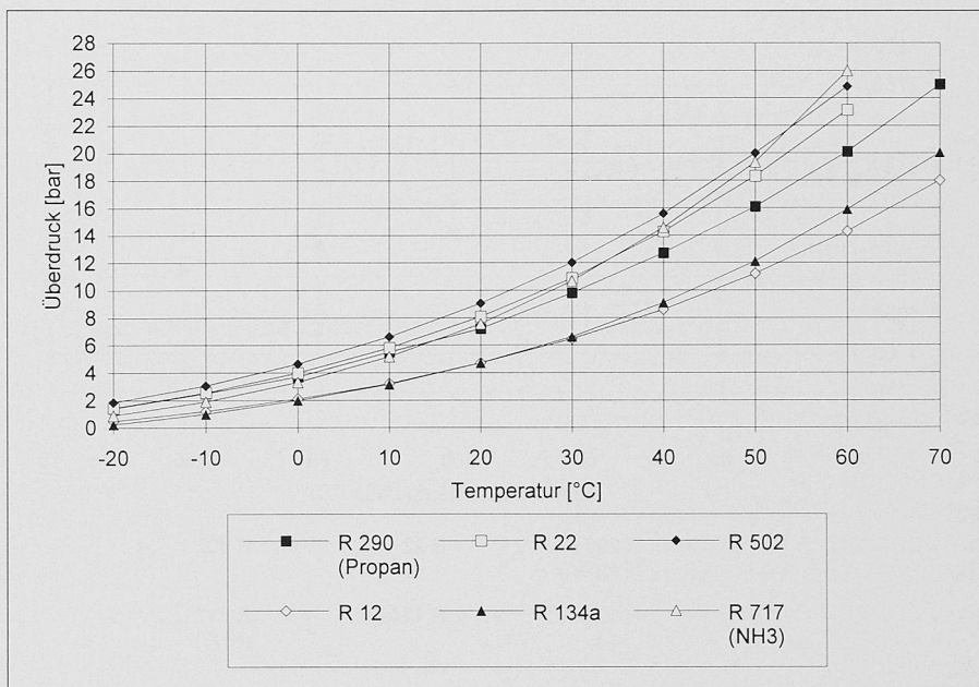
Bild 1. Dampfdruckkurven
