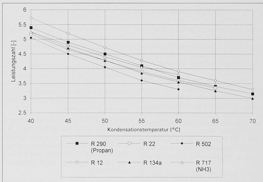
Bild 3. Leistungszahlen, Verdampfungstemperatur, t_0 = -10^\circ\text{C} , isentrope Verdichtung
